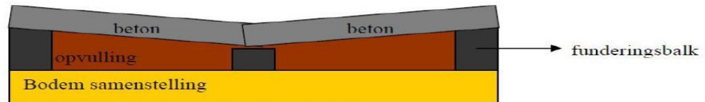
Fundering Zijaanzicht Centrale Bunkercomplex
